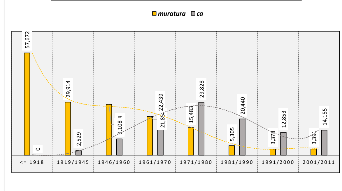
NUMERO EDIFICI PER EPOCA DI COSTRUZIONE E TIPOLOGIA STRUTTURALE
